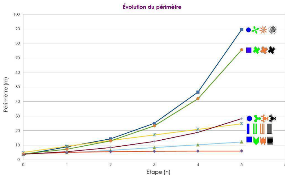
Figure 32 - Comparaison 2 de périmètres
